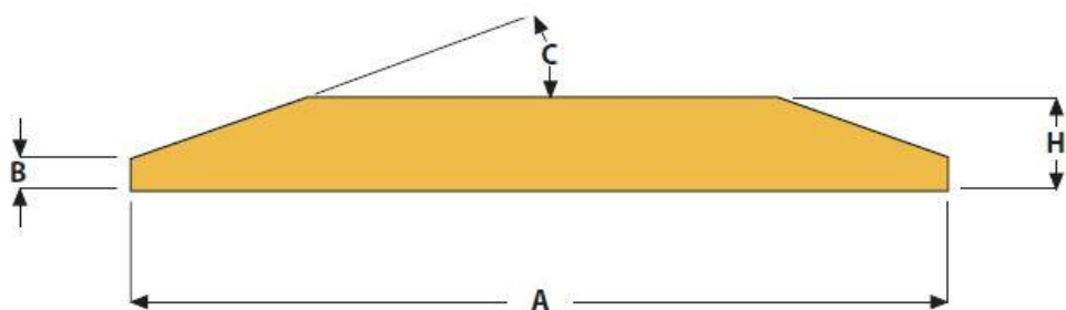
Tabulka břitů s oboustranným úkosem
