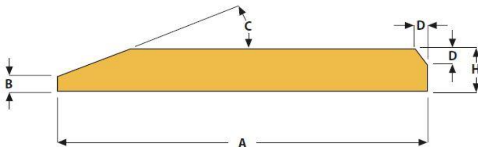
Tabulka břitů s jednostranným úkosem
